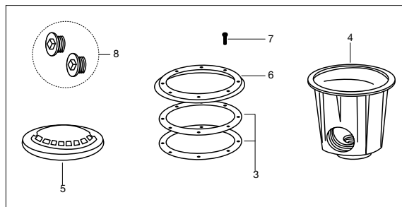
Refacciones dren de fondo MD
