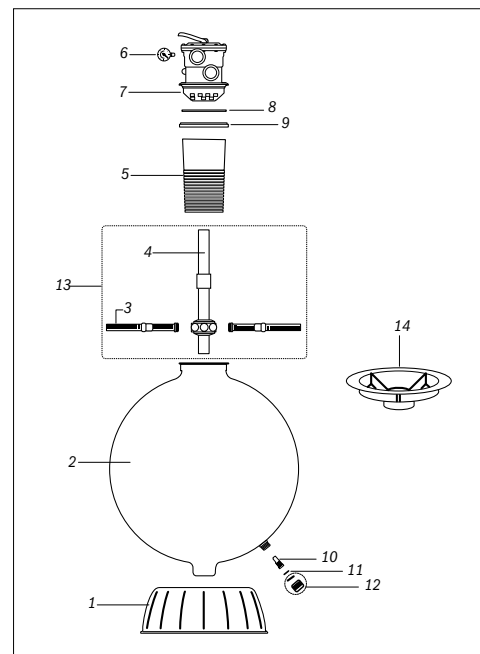
Esquema de partes filtro Sand Storm
