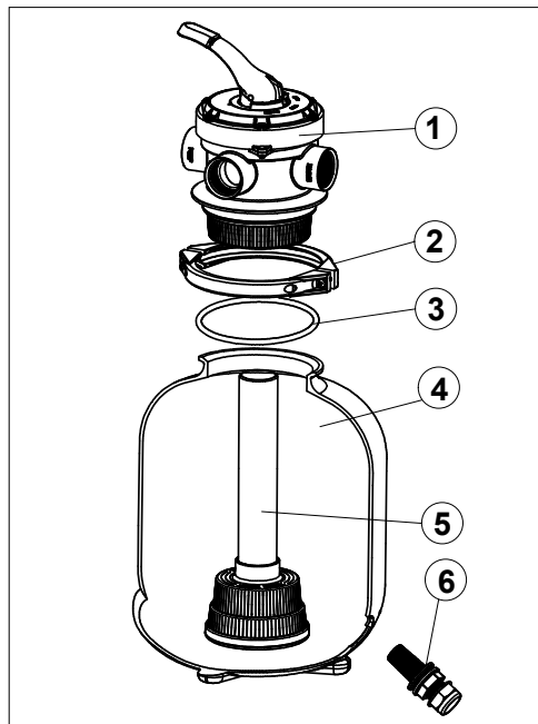
Esquema de partes filtro Pacific 14"
