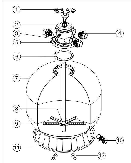
Esquema de partes filtro Indian (28")
