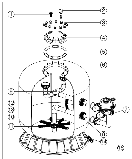
Refacciones filtro Atlantic (28", 32" y 36")
