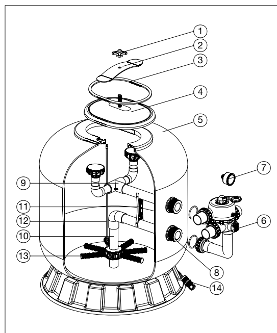
Refacciones filtro Atlantic (40")
