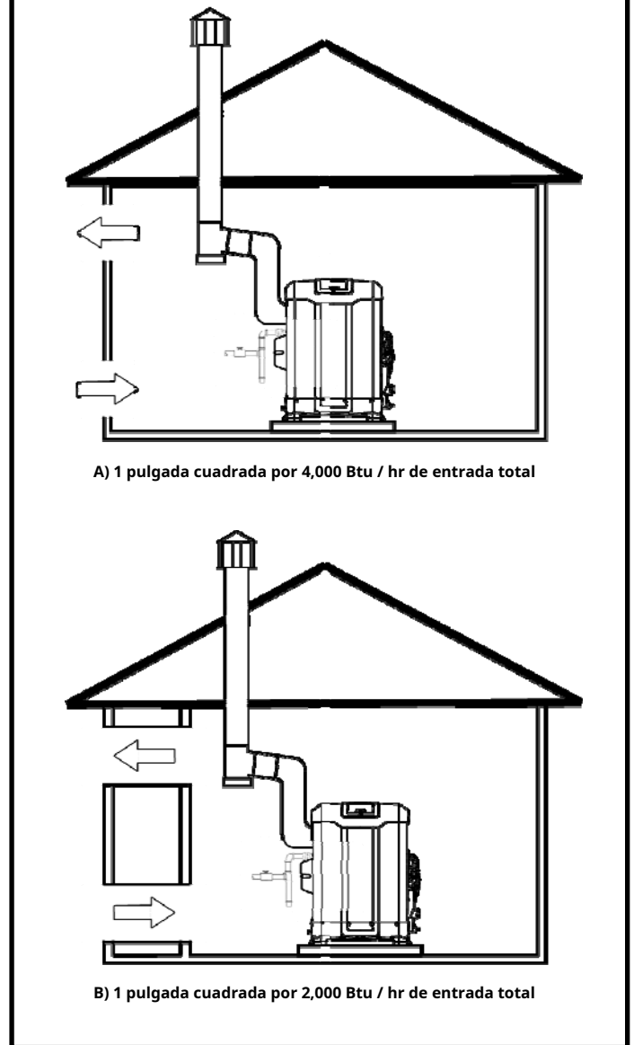
Figura 8: Instalación de aire procedente del exterior del edificio
