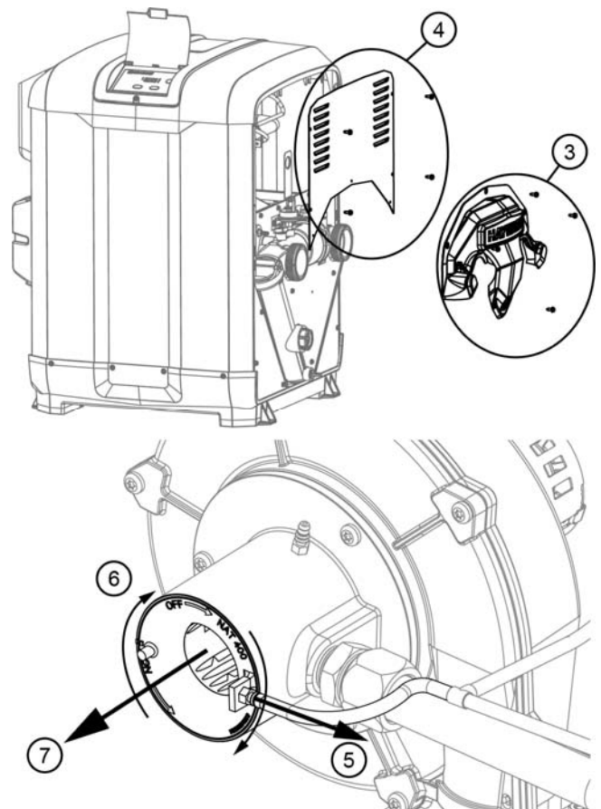
Figura 6: Extracción del mezclador de aire / combustible
