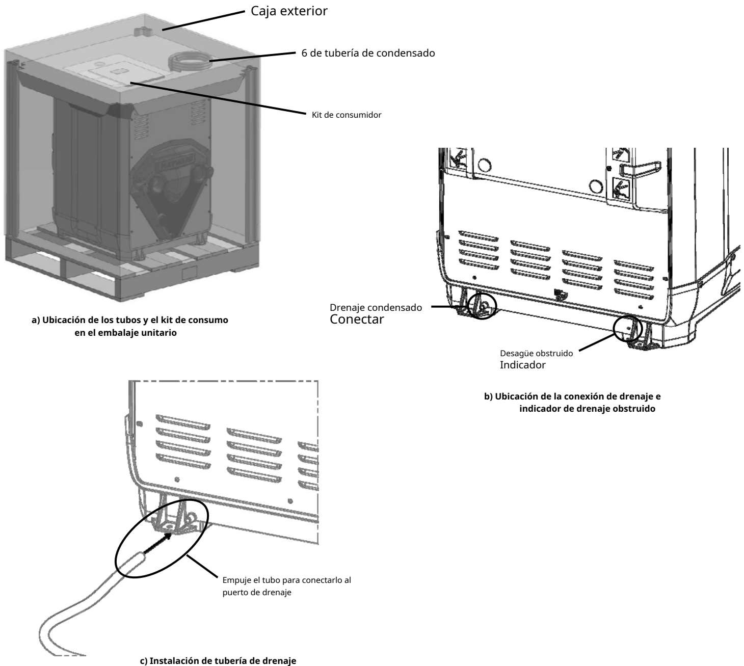
Figura 5: Instalación del drenaje de condensado
