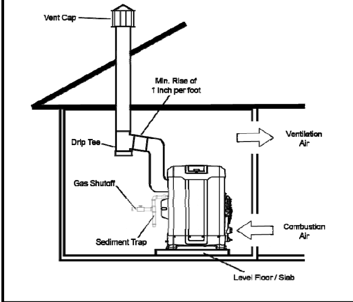
Figura 7: Instalación de aire procedente del interior del edificio 1 pulgada cuadrada por 1000 Btu / h de entrada total
