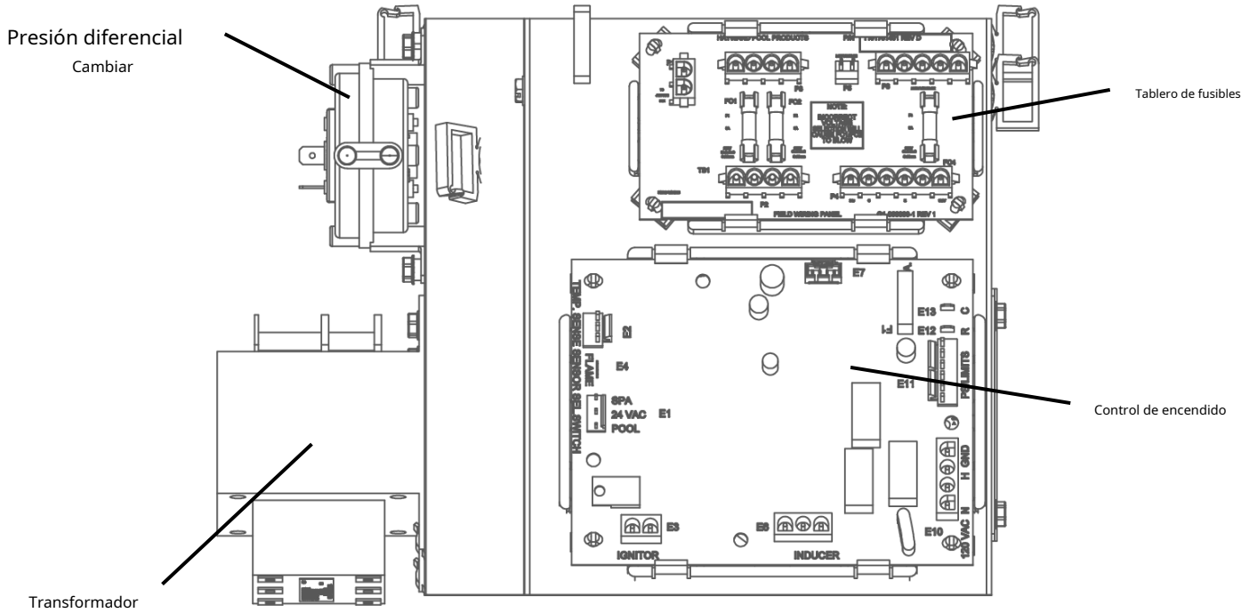
Figura 21: Componentes del ensamblaje del encabezado
