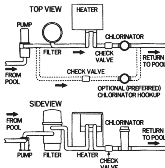
Figura 18: Clorador automático
