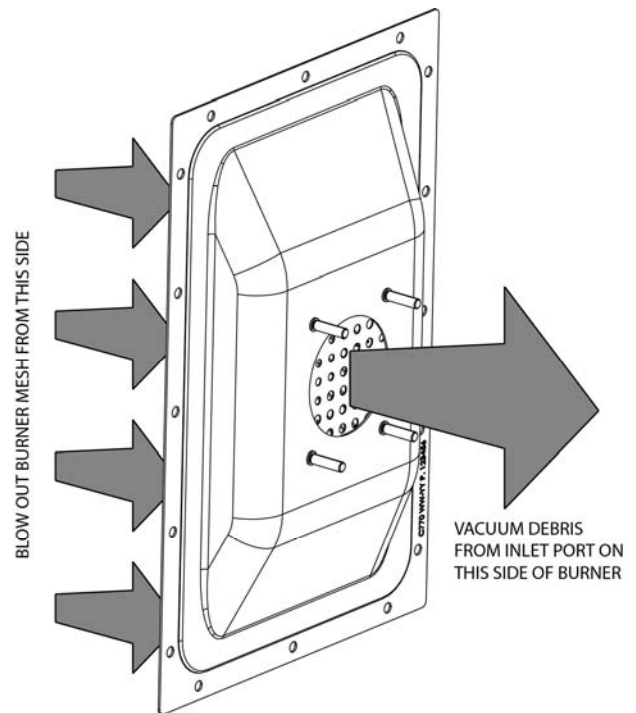
Figura 29: Limpieza del quemador
