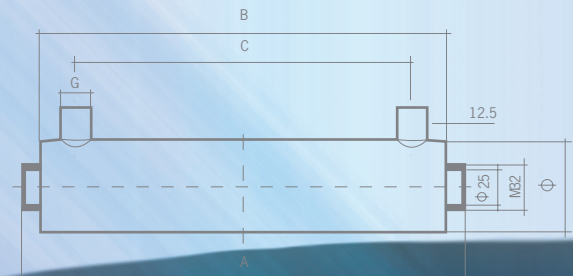
Esquema de dimensiones para lámparas entre 16 y 165 W
