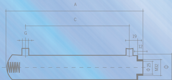
Esquema de dimensiones para lámparas entre 4 y 12 W
